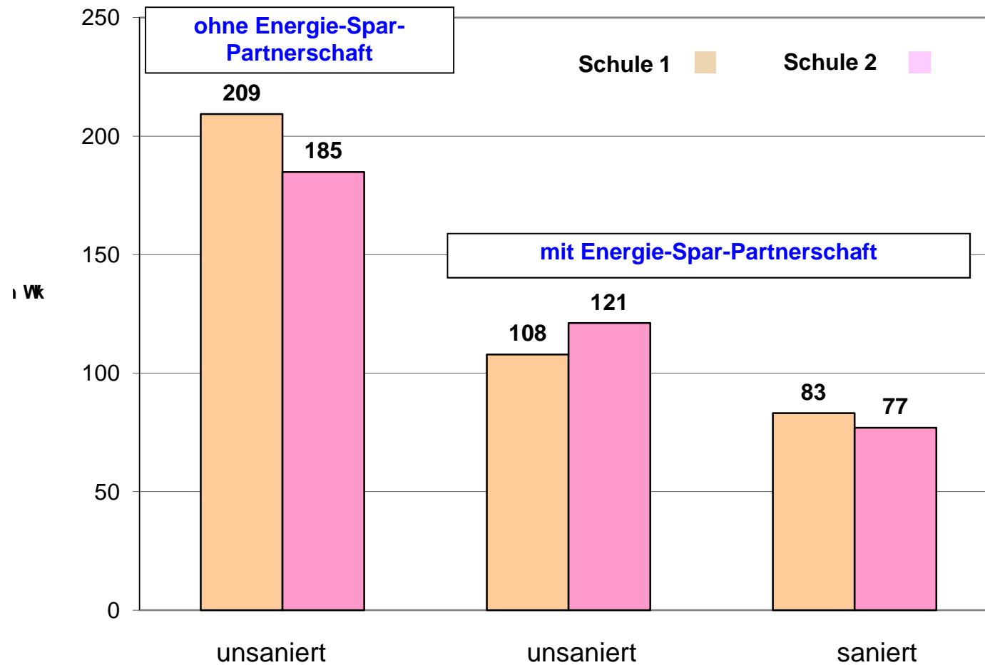
Entwicklung des Wärmeverbrauchs von zwei Schulen des Typs Erfurt am Standort Erkner
